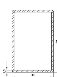
nr: 90-235-15 Armatura pentru cercevea usa Усилитель створки дверной
