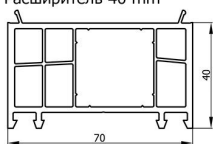
nr: 7151 Inaltare/latire rama 40 mm Расширитель 40 mm
