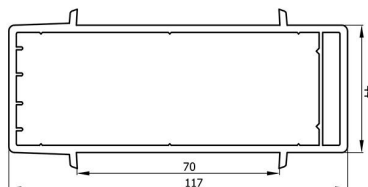
nr: 7156 Imbinare statica pt fatada 44 mm Соединитель статический фасадный
