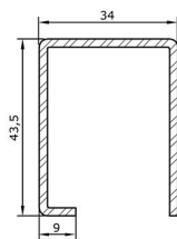
nr: 90-243-15 Armatura pentru cercevea usa balcon Усилитель створки балконной
