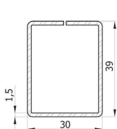
nr: 90-232-15 Armatura pt toc usa Усилитель для рамы дверной
