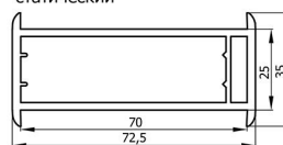
nr: 7156 Imbinare statica pt fatada 44 mm Соединитель статический фасадный
